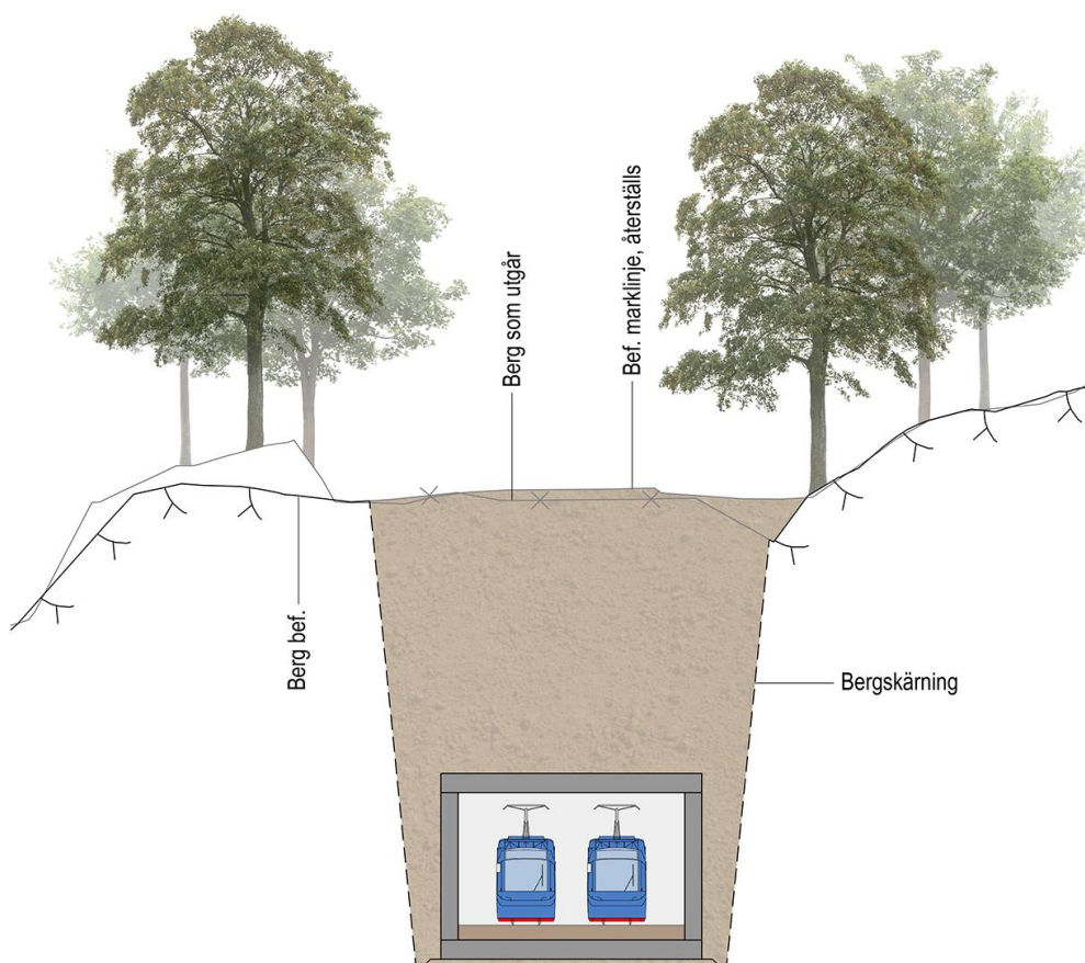
Figur 13. Principsektion genom tunneln där den nått södra sidan av Roslagsvägen. Berglacken mot vägen och träden som växer där avses sparas. Ur gestaltungsprogrammet.
