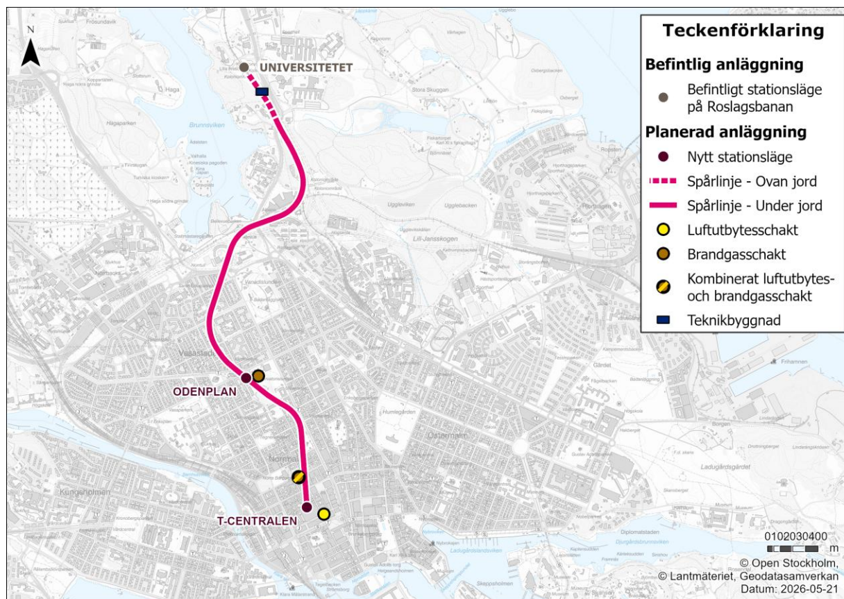
Figur 14. Placering av anläggningar ovan jord längs den nya sträckningen av Roslagsbanan.
