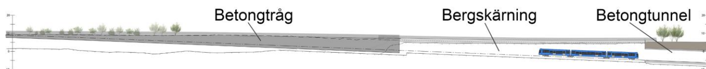
Figur 10. Längdprofil för betongtråget, bergschaktet och tunnelmynningen sett från väster. Ur gestaltningsprogrammet.
