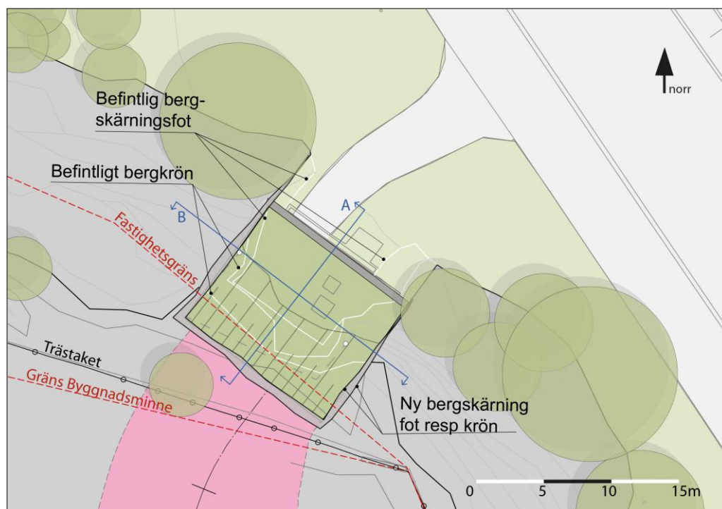
Figur 53. Illustration ur gestaltningsprogrammet. Plan vid tunnelmynningen för Arbetstunnel Bellevue. (Observera att utformningen inte avgörs i järnvägsplanen, bilden visar endast en möjlig lösning.)
