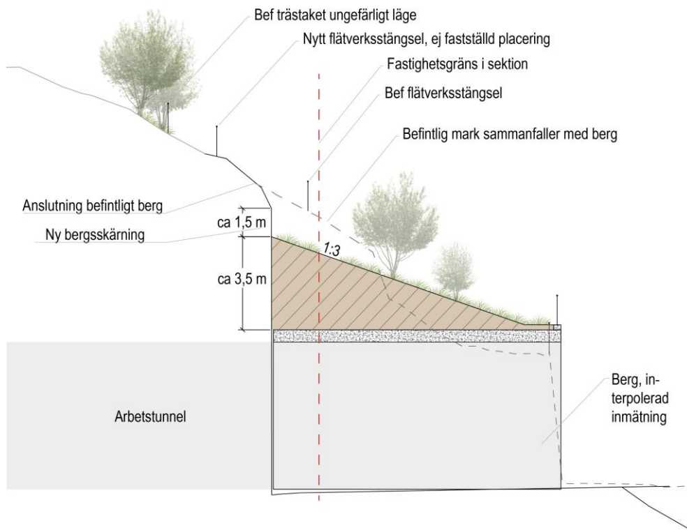
Figur 55. Sektion genom berg och port för Arbetstunnel Bellevue. (Observera att utformningen inte avgörs i järnvägsplanen, bilden visar endast en möjlig lösning.)
