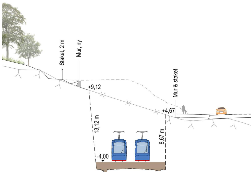
Figur 12. Principsektion vid bergschaktet strax norr om betongtunnelmynningen. Gång- och cykelbanan på Roslagsvägens södra sida till höger i bild. Ur gestaltungsprogrammet.
