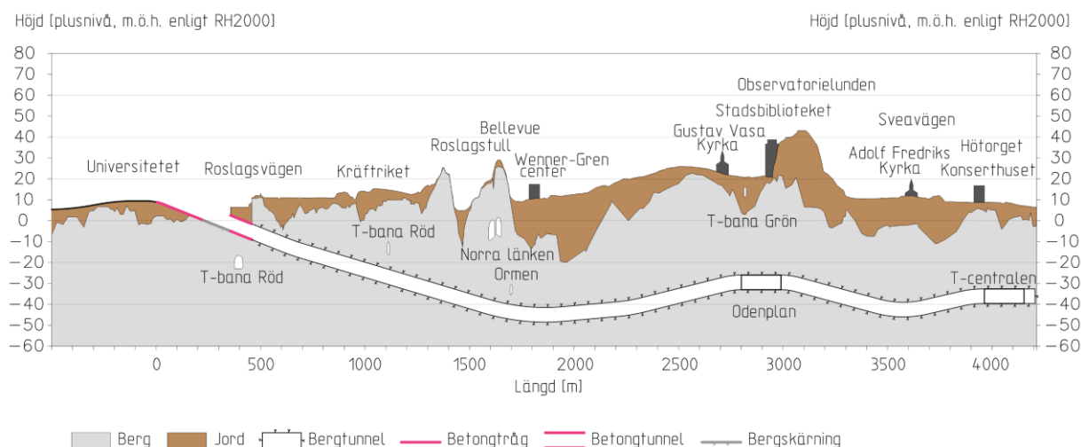
Figur 9. Illustrativ spårprofil som visar norr till vänster och söder till höger. I figuren syns även målpunkter ovan jord samt befintliga underjordsanläggningar.
