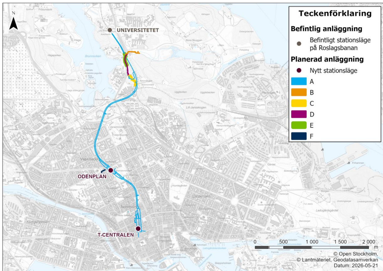
Figur 16. VA-lösningar för anläggningen, som i vissa delar utgör alternativ till varandra. A är tunnelsystemets tunnelvattenledningar, B är vattenledning i Lilla Frescati, C är vattenledning som ansluter till befintlig eller planerad dagvattenkanal i Albano, D är en ny vattenledning längs Roslagsvägen, E och F är alternativ med korta anslutningsledningar till befintliga vattenledningar.
