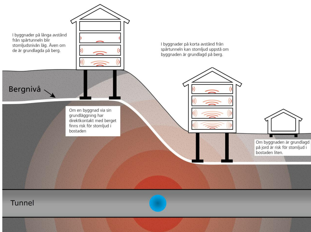
Figur 73. Vibrationsutbredning i berg från ljudkälla som skapar stomljud i byggnader. Ljudkällan anges med blå cirkel i figuren.
