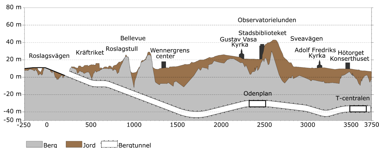
Figur 2. Illustration över spårlinjens profil.
