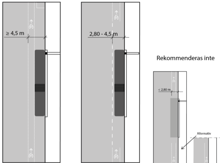
Figur 33 Exempel på utformning av cykelfält vid busshållplats.
