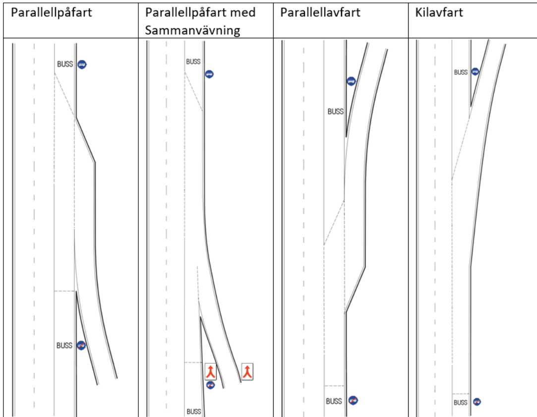
Figur 10 Principutförning av busskörfält förbi på- och avfarter.
