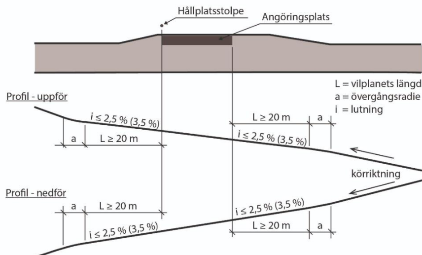
Figur 48 Vilplan vid hållplatsläge.
